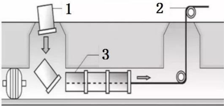
图 7 短管内衬法修复原理示意图
