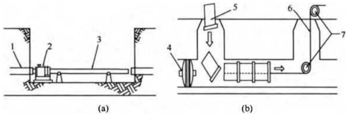
图 2 不连续穿插法示意图
